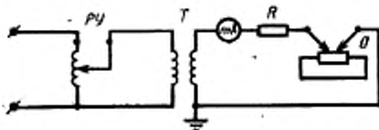
ПУ—регулирующее устройство; Т—трансформатор; R—сопротивление 0,5 МОм; B—образец из карболита с нанесенной пленкой испытуемой эмали.
