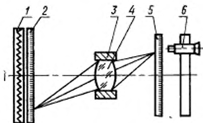
1—осветитель шкалы; 2—шкала в предметной плоскости; 3—объективодержатель; 4—испытуемый объектив; 5—шкала в плоскости изображений; 6—микроскоп.
