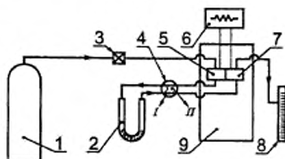
1 — баллон с газом-носителем; 2 — U-образная трубка; 3 — вентиль тонкой регулировки; 4 — четырехходовой кран; 5 — сравнительная ячейка детектора; 6 — самописец; 7 — измерительная ячейка детектора; 8 — измеритель скорости газ-носителя; 9 — термостат
