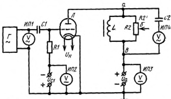
R1, R2 —резисторы; C1, C2 —конденсаторы; L —дроссель; L —испытываемая лампа; ИП1, ИП4—вольтметр переменного тока; ИП2, ИП3—вольтметры постоянного тока; G —генератор синусоидального напряжения.
