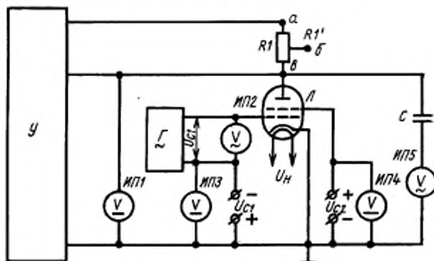
R1 —резистор; C —конденсатор; L —испытуемая лампа; ИП1 , ИП3 , ИП4 —вольтметры постоянного тока; ИП2 , ИП5 —вольтметры переменного тока; Г —генератор синусоидального напряжения; У —источник питания анода, непосредственно стабилизирующий напряжение анода.
