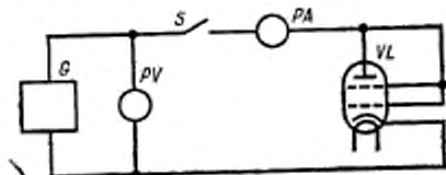
PV—вольтметр постоянного тока; PA—миллиамперметр постоянного тока; S—выключатель; VL—испытываемая лампа; G—источник напряжения постоянного тока.
