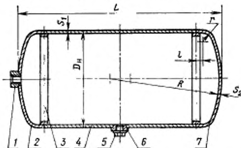
1—штуцер дна; 2—днше с отверстием; 3—кольцо подкладное; 4—обечайка; 5—пробка; 6—штуцер обечайки; 7—днше глухое.
