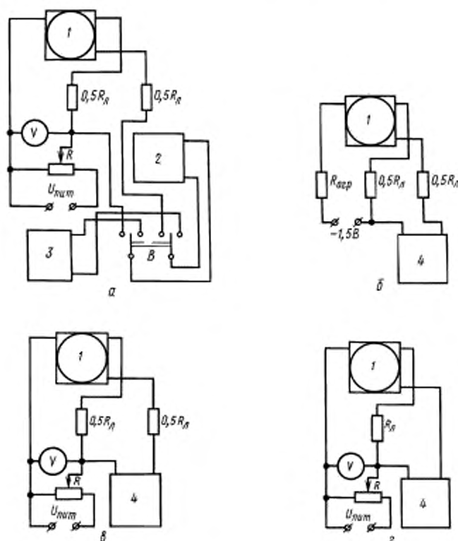
Схемы подключения логометров к внешней цепи
