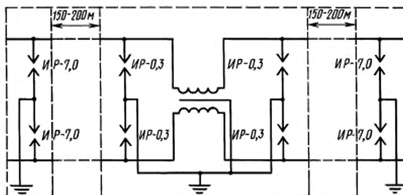
Защита пупиновских катушек
