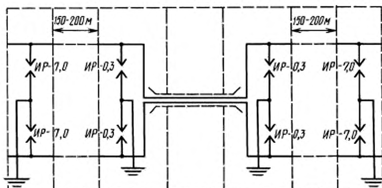
Защита кабельных вставок
