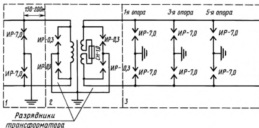
1 — фидерная линия; 2 — абонентский трансформатор; 3 — абонентская линия
