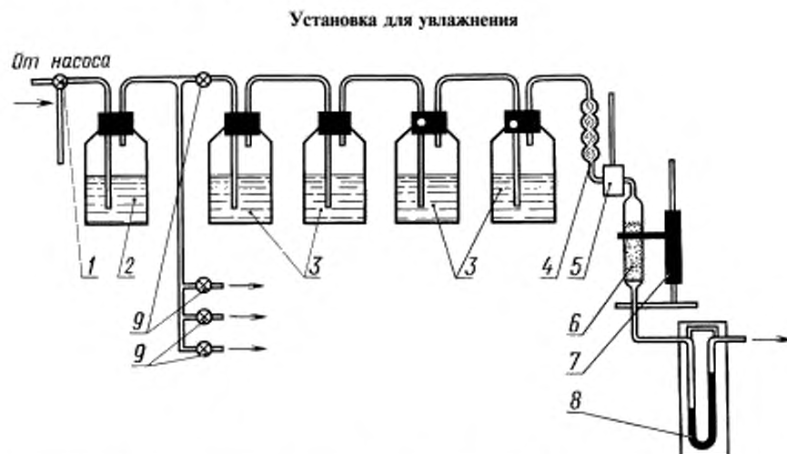
1 — трехходовой кран; 2 — склянка с водой; 3 — склянка с кислотой; 4 — брызгоуловитель; 5 — карман с термометром; 6 — динамическая трубка; 7 — штатив; 8 — реометр; 9 — двухходовые краны
