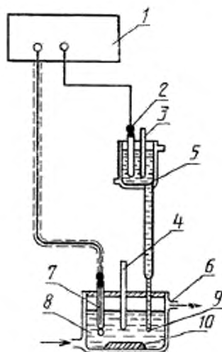
Схема измерения потенциала электрода
