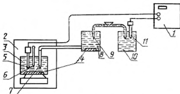
Схема измерения потенциала электрода при минусовых температурах
