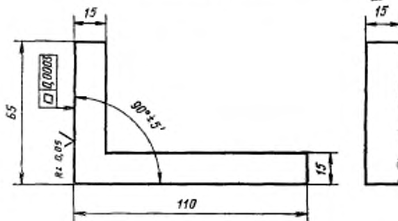
Специальный угольник
