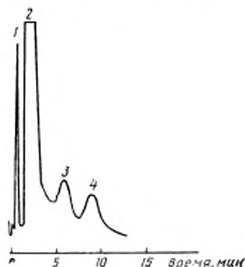
1—этиленгликоль; 2—диэтиленгликоль; 3—дециловый спирт; 4—триэтиленгликоль
