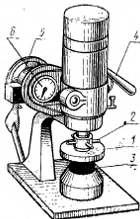
1 — патрон, 2 — гайка; 3 — подушечка, 4 — рукоятка, 5 — мотор; 6 — счетчик.
