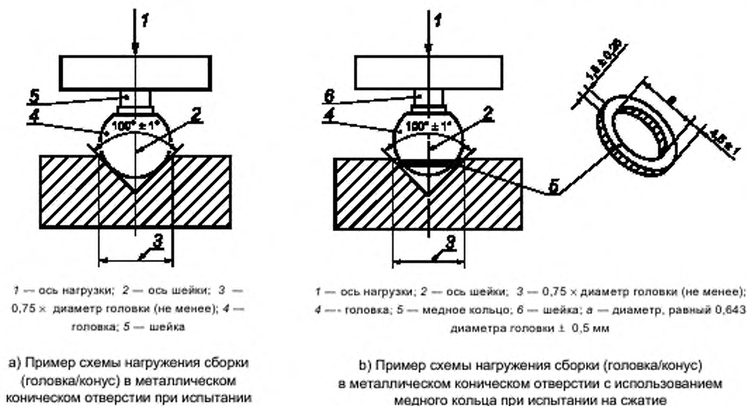
Рисунок 3 — Пример схемы нагружения сборки (головка/конус) в металлическом коническом отверстии
