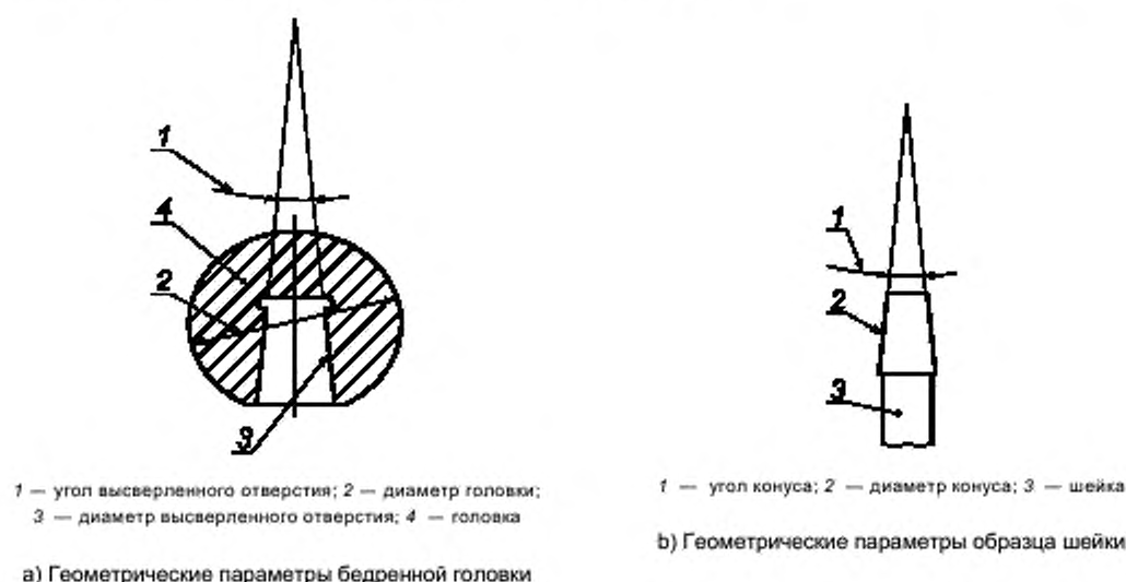
Рисунок 1 — Геометрические параметры соединения головки и шейки
