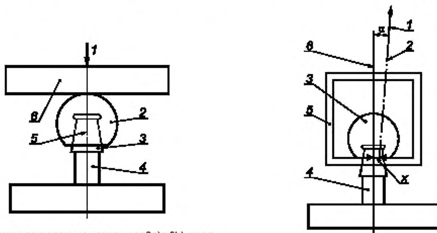
Рисунок 3 — Пример схемы нагружения сборки (головка/конус) в металлическом коническом отверстии
