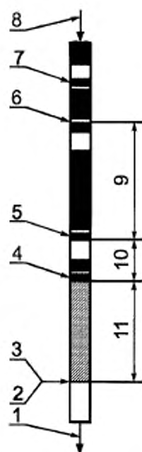
1 — нижняя часть; 2 — фронт элюирования; 3 — чистая жидкость; 4 — первая интенсивная желтая флуоресценция; 5 — первая интенсивная голубая флуоресценция; 6 — красное кольцо; 7 — дополнительное красное кольцо; 8 — верхняя часть; 9 — зона ароматики; 10 — зона олефинов; 11 — зона насыщенных углеводородов
