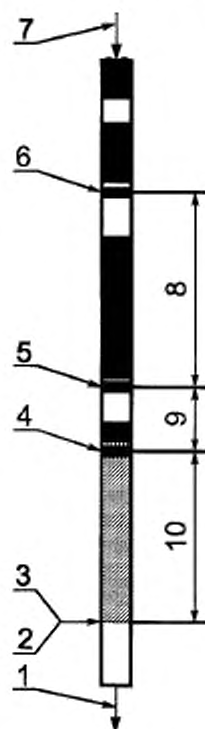
1 — нижняя часть; 2 — фронт элюирования; 3 — чистая жидкость; 4 — первая интенсивная желтая флуоресценция; 5 — первая интенсивная голубая флуоресценция; 6 — красное кольцо; 7 — верхняя часть; 8 — зона ароматических углеводородов; 9 — зона олефинов; 10 — зона насыщенных углеводородов
