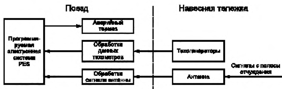
Рисунок В.2 — Блок-схема системы АТЗ
