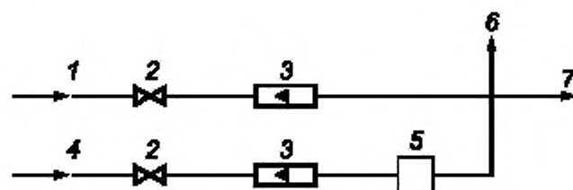
1 — ввод калибровочного газа, содержащего NO; 2 — клапан тонкой регулировки; 3 — расходомер; 4 — ввод кислорода; 5 — генератор озона (регулируемый); 6 — сброс излишка испытательного газа; 7 — подача испытательного газа в конвертер и на вход газоанализатора
