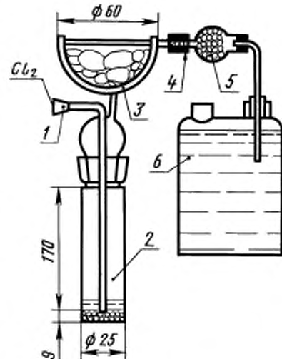
1 — штатив; 2 — пробирка с навеской олова и четыреххлористым углеродом; 3 — доушка, охлаждаемая льдом; 4 — трубка резиновая; 5 — трубка с хлористым кальцием; 6 — склянка со щелочью (10 %-ный раствор) для поглощения избытка хлора
