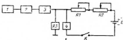
1—поверяемый генератор; 2—измерительный аттенюатор; 3—детекторная головка; 4—фотокомпенсационный микровольтмикроамперметр типа Ф 116/2; R1 , R2 —переменные резисторы типа СП1; R3 —резистор 3 кОм, 0,5 Вт; K —ключ; E —источник постоянного тока.
