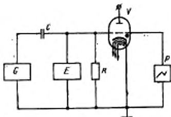
C — переходной конденсатор; E — фильтр; G — источник импульсного напряжения; P — осциллограф; R — резистор утечки; V — испытываемый тиристор
