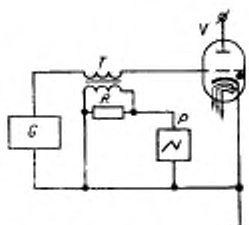
Г — источник импульсного напряжения; Р — осциллограф; T — измерительный трансформатор тока; R — резистор; V — испытываемый тиратрон
