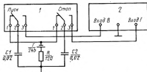
Г — поверяемый прибор; 2 — электронно-счетный частотомер; C1 и C2 — электрические постоянные конденсаторы; P — постоянный резистор; G — источник постоянного тока.
