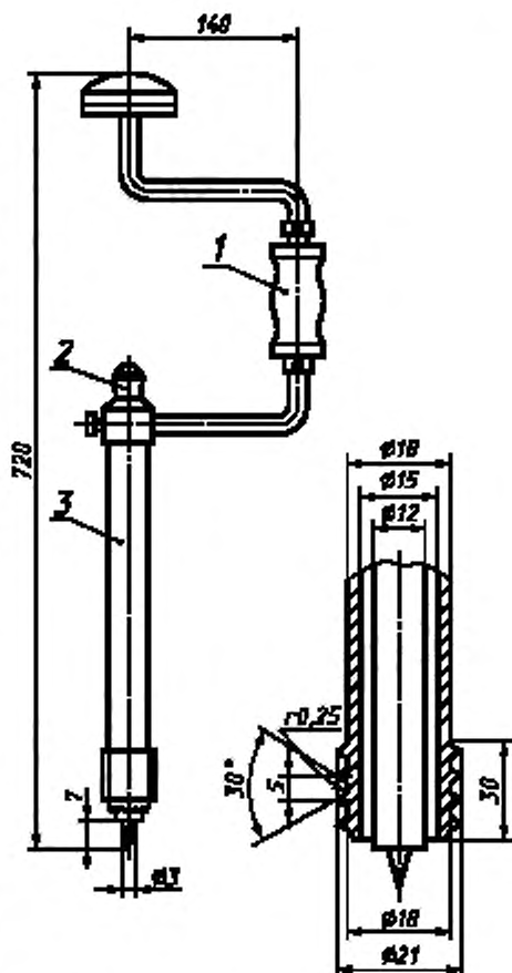
1 — коловорот; 2 — толкатель, 3 — бур
