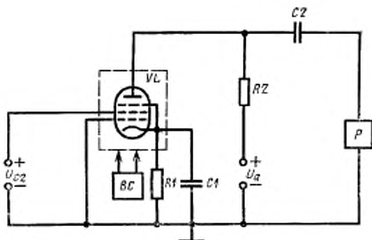
P —электронный вольтметр или регистрирующее (запоминающее) устройство; R1 , R2 —резисторы; C1 , C2 —конденсаторы; BC —вибрационный стенд; VL —испытуемая лампа
