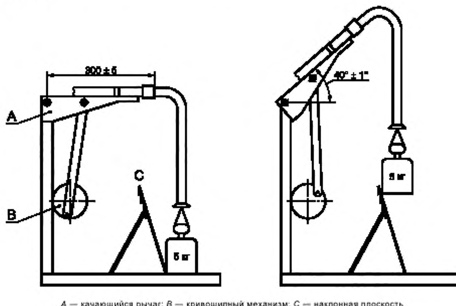
А — качающийся рычаг; В — кривошипный механизм; С — наклонная плоскость
