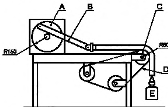
A — кривошипный механизм; B — соединительный стержень, C — ролик диаметром 120 мм, D — ролик из абразивной ленты; E — груз
