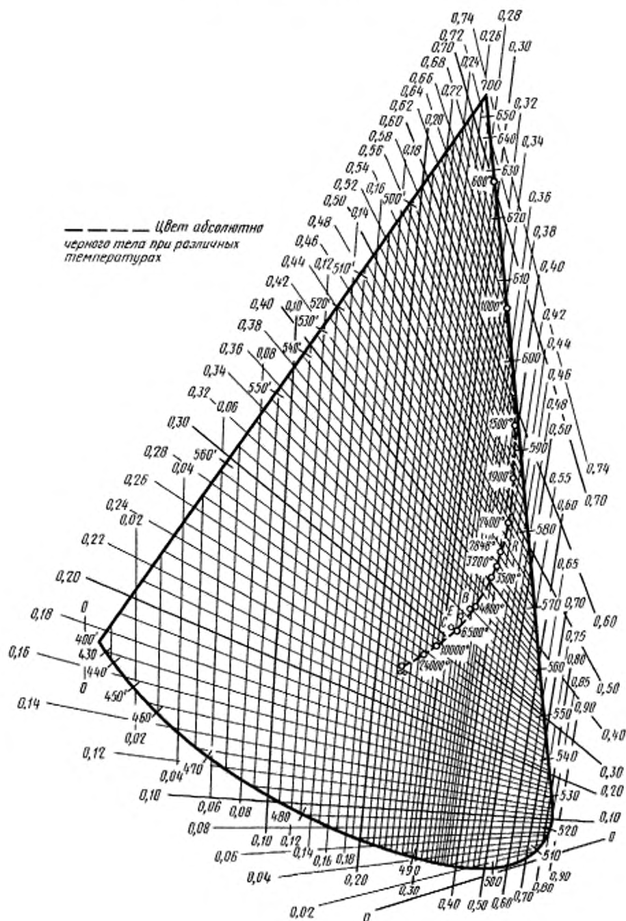
Равноконтрастный цветовой график
