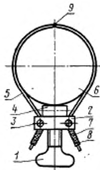
1—винт; 2—плата; 3—установочный винт; 4—шайба; 5—термоэлектроды; 6—лампа; 7—чулок из стеклянного волокна; 8—изоляция; 9—точка сварки термоэлектродов.
