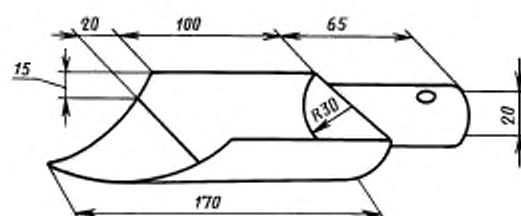
Щуп для отбора точечных проб
