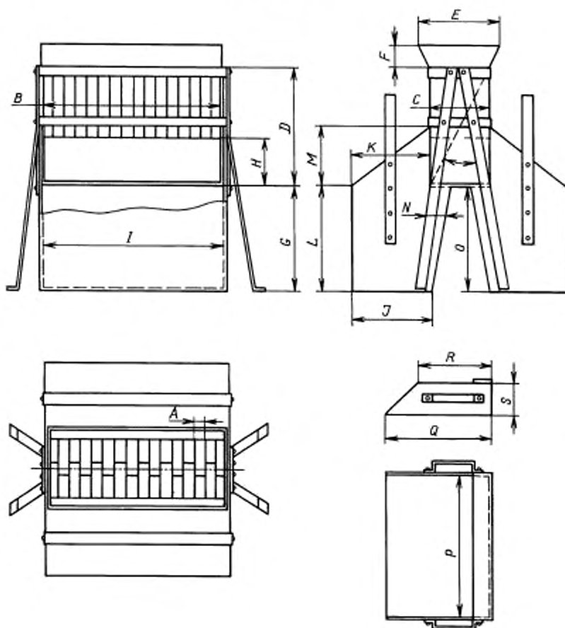
Делитель желобчатый
