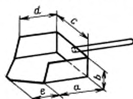
Совок для отбора точечных проб
