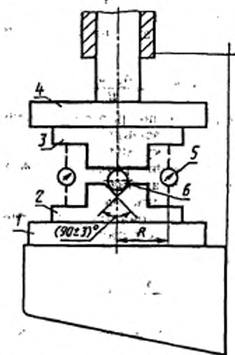
1 и 4 — плиты; 2 и 3 — стальные призмы; 5 — индикатор; 6 — шарик
