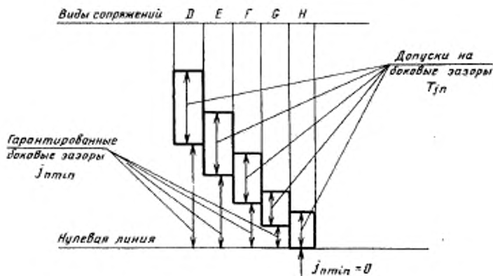
Виды сопряжений и гарантированные боковые зазоры
