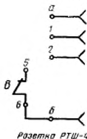
Электрическая принципиальная схема
