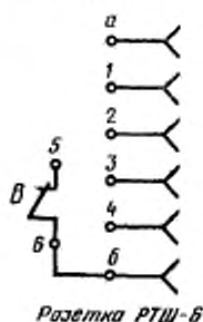
Электрическая принципиальная схема
