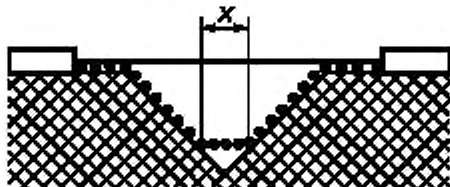
Рисунок F.2 — Широкая канавка
