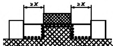
Рисунок F.5 — Несплошной стык с узкими канавками
