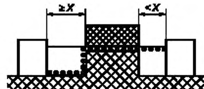
Рисунок F.6 — Несплошной стык с широкими канавками
