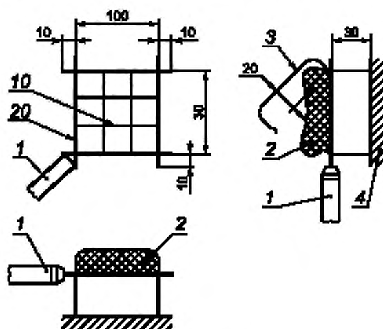
1 — ручка; 2 — ватный тампон; 3 — зажим; 4 — поверхность опытного образца
