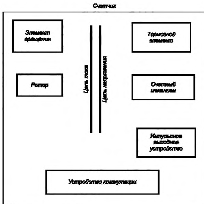
Рисунок С.1 — Структурная схема электромеханического счетчика
