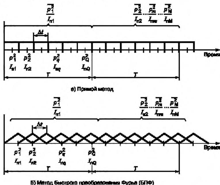
Рисунок 3 — Вычисление усредненных по времени интенсивностей звука \overline{I_{nm}} и квадратов звукового давления \overline{p_m^2} , m = 1, 2, 3, \dots, M на времени усреднения T по измеренным последовательным значениям интенсивности I_{nQ} и квадрату звукового давления p_Q^2
