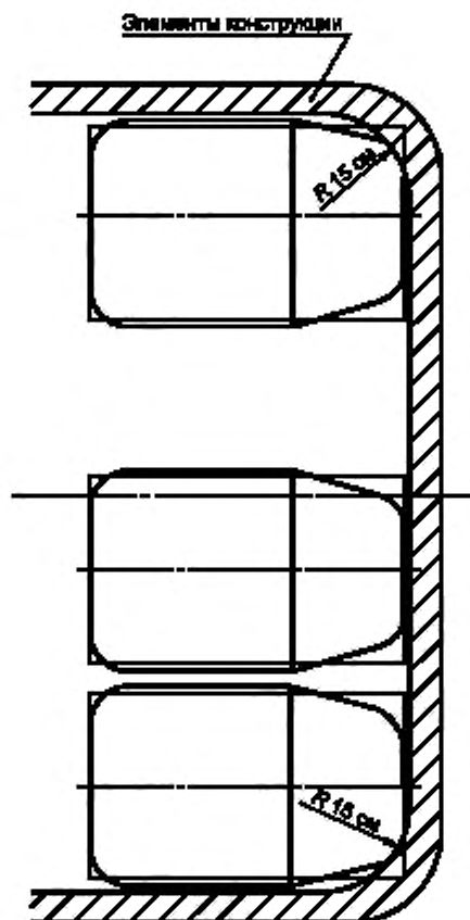
Рисунок 11 — Допустимое выступание конструкции в зону задних боковых сидений. Вид в плане зоны, предназначенной для размещения сидений (два задних боковых сиденья) (см. 5.7.8.1.4)
