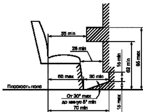
Рисунок 16 — Пространство для сидящих пассажиров (см. 5.7.8.5)
