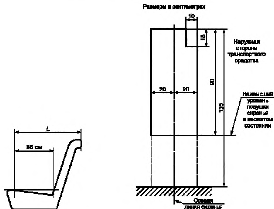
Рисунок 5 — Длина зоны, предусмотренной для сиденья (см. 5.7.8.1.1)
