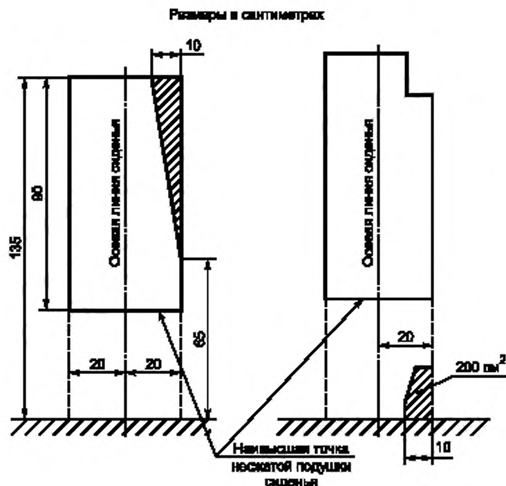
Рисунок 7 — Допустимое выступание деталей конструкции внутрь зоны сиденья. Определение треугольной зоны, в которую может выступать элемент конструкции (см. 5.7.8.1.3.2)
