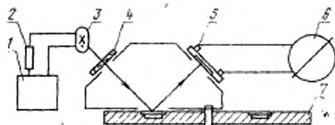
1—стабилизатор напряжения В 2-2; 2—дроссели; 3—бал- ласт; 4—ртутная лампа ДБ-18; 4—стеклянная пластинка, не пропускающая излучение с длиной волны 253,7 нм, 5—фо- тоэлемент селеновый с корректирующим фильтром ФЭС-10, 6—гальванометр типа М 1952; 7—поворотный диск с кю- ветами для люминофора
