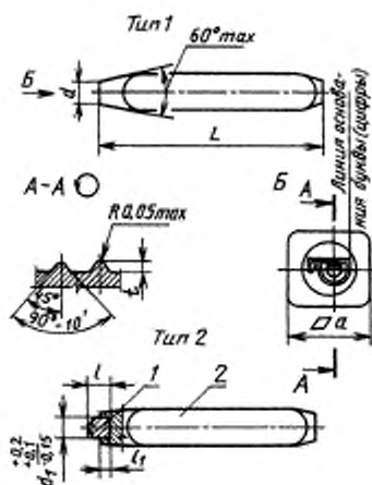
1 — вставка; 2 — державка
