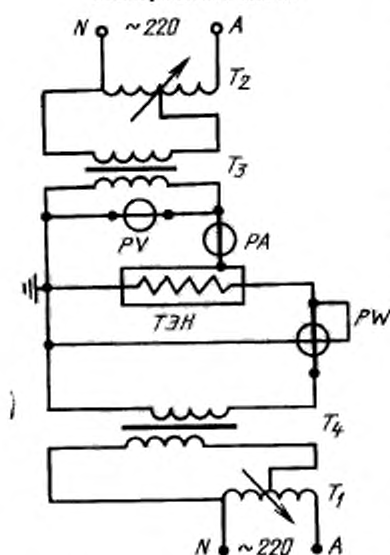
Электрическая схема
