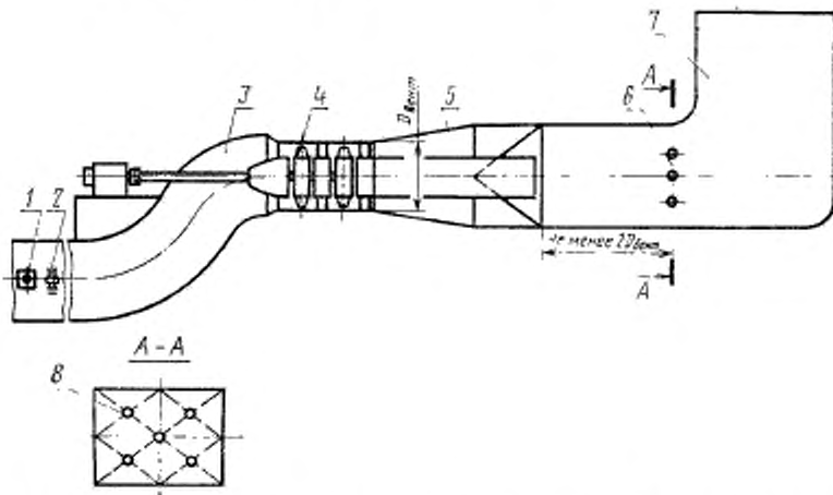
1—датчики давления вентилятора; 2—датчики подачи вентилятора; 3—канал вентилятора; 4—вентилятор; 5—диффузор; 6—измерительная поверхность; 7—выходная часть; 8—точки измерения
