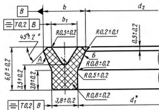
Манжеты для уплотнения цилиндров диаметром D = 12 - 22 мм и штоков диаметром d = 4 - 14 мм (черт. 1, табл. 1)
