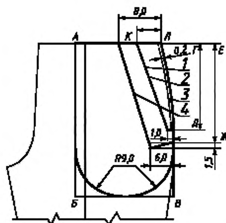
1 — край верхней части подкладки бокового кармана; 2 — линия перегиба бокового кармана и среза подкладки; 3 — подкладка в боковой карман; 4 — подзор бокового кармана
