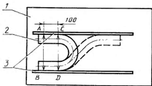
1—контрольная плита; 2—изделие; 3—проверочные линейки
