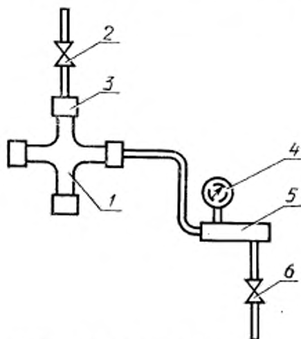
1—изделие; 2—кран для выпуска воздуха; 3—заглушка; 4—манометр; 5—насос; 6—кран для подачи воды
