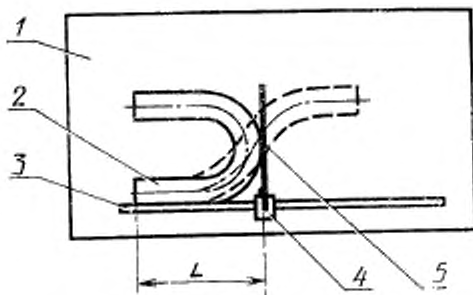
1—контрольная плита; 2—изделие; 3—контрольная линия; 4—ползун; 5—упор
