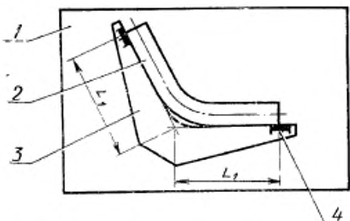
1—контрольная плита; 2—изделие; 3—щуп; 4—поле допуска
