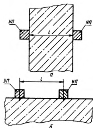
а — схема испытания бетона способом сквозного прозвучивания; б — схема испытания бетона способом поверхностного прозвучивания; УП — ультразвуковые преобразователи, l — база прозвучивания
