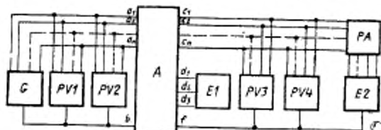
G —источник постоянного и переменного напряжений; PV1 —измеритель постоянного напряжения; PV2 — измеритель переменного напряжения; A —НСН; a_1, a_2, \dots, a_n , b —входы НСН; c_1, c_2, \dots, c_n , f —выходы НСН; d_1, d_2, d_3 —выводы подключения обратной связи; E1 —блок делителей; PV3 —измеритель постоянного напряжения; PV4 —измеритель переменного напряжения; PA —измеритель постоянного тока; E2 —блок нагрузок НСН
