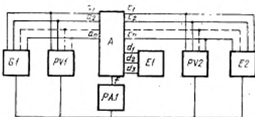
G1 — источник постоянного напряжения; PV1 , PV2 — измерители постоянного напряжения; A — НСН; a_1, a_2, \dots, a_n — входы НСН; c_1, c_2, \dots, c_n — выходы НСН; d_1, d_2, d_3 — выходы подключения обратной связи; f — общий вывод; PA1 — измеритель постоянного тока; E1 — блок делителей; E2 — блок нагрузок НСН
