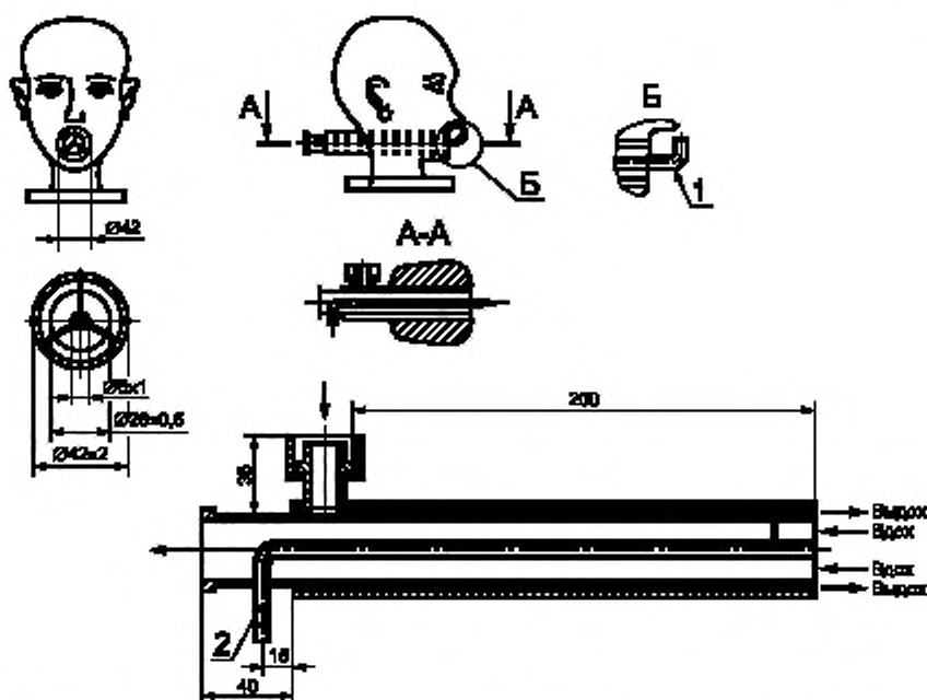
1 — штука для измерения сопротивления воздушному потоку; 2 — измерение CO 2 (на входе)
