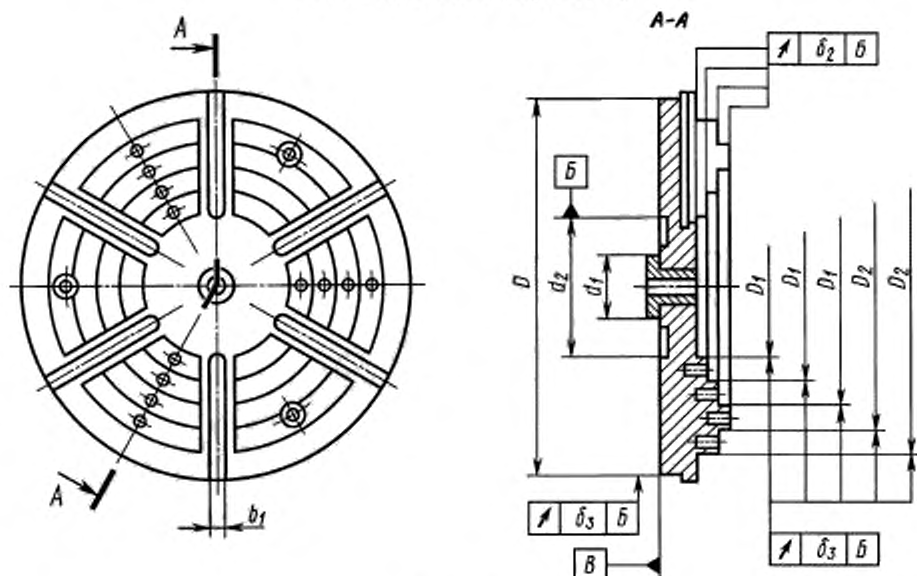
Планшайбы плоские (черт. 37, 38)
