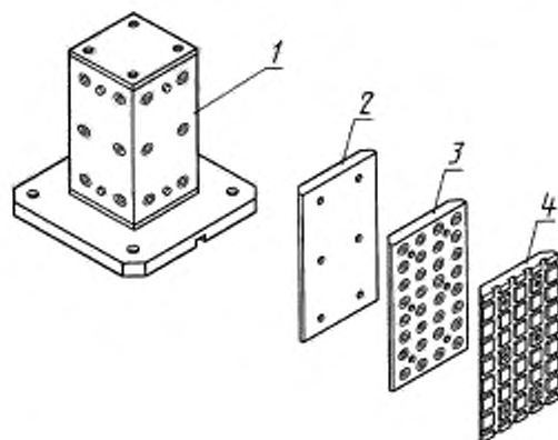
Схема переконфигурации корпусной части приспособления типа «четырёхсторонняя стойка»
