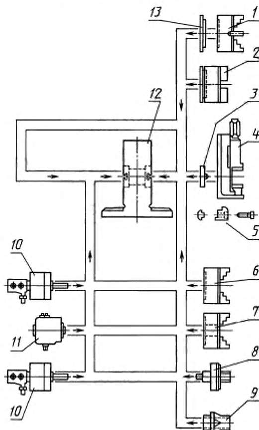
Схема переконфигурации корпусной части приспособления типа «двухсторонняя стойка»
