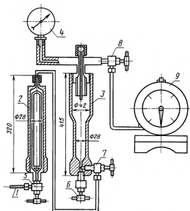
1 — вход газа; 2 — фильтр-патрон; 3 — абсорбирующий сосуд; 4 — манометр; 5, 6, 7, 8 — запорные вентили; 9 — газовый счетчик
