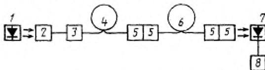
1—источник излучения; 2—устройство ввода; 3—смеситель мод; 4—вспомогательное оптическое волокно; 5—оптические разъемные соединители; 6—измеряемый кабель; 7—приемник излучения; 8—регистрирующее устройство
