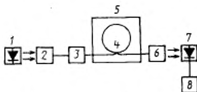
1—источник излучения; 2—устройство ввода; 3—смеситель мод; 4—измеряемый кабель; 5—камера внешних воздействий; 6—фильтр мод оболочки; 7—приемник излучения; 8—регистрирующее устройство
