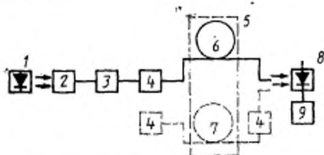
1—источник излучения; 2—устройство ввода; 3—смеситель мод; 4—фильтр мод оболочки; 5—измеряемый кабель; 6—оптическое волокно, подверженное влиянию; 7—влияющее волокно; 8—приемник излучения; 9—регистрирующее устройство
