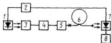
1—источник излучения; 2—блок управления; 3—устройство ввода; 4—смеситель мод; 5— фильтр мод оболочки; 6—измеряемый кабель; 7—приемник излучения; 8—регистрирующее устройство
