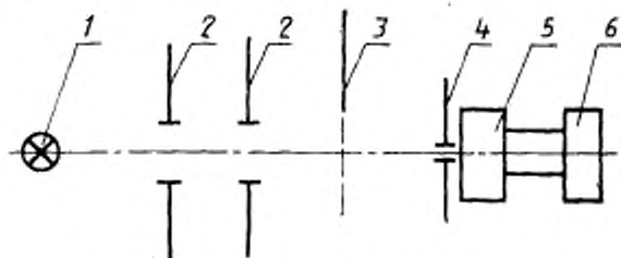
1—рабочая светозмерительная лампа или лампа, для которой определяется спектральный коэффициент; 2—светозащитная диафрагма; 3—заслонка; 4—диафрагма с калиброванным отверстием; 5—приемник излучения; 6—измерительный прибор
