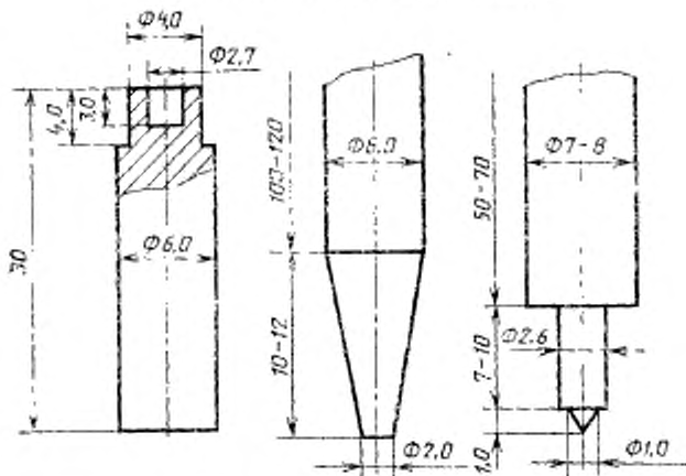
Нижний электрод
