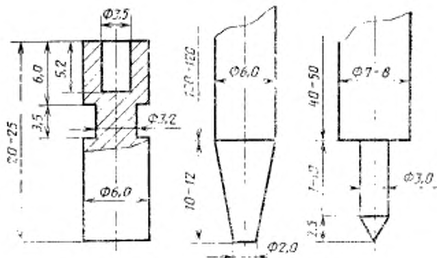
Нижний электрод
